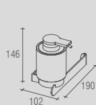
BA 0243 - Miss by Zen Saboneteira líquida fixa com papelreira
