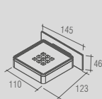
BA 0161 - Supreme Saboneteira fixa com acrílico removível
