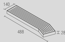
BA 0526 - Soho Prateleira com saboneteira
