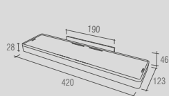
BA 0164 - Supreme Prateleira de acrílico
