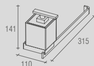
BA 0265 - Be Saboneteira líquida fixa com toalheiro
