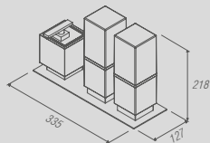
PR 0052 - Oriente Stone Saboneteira líquida e porta objetos de balcão
