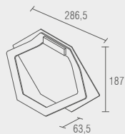
BA 0603 - Elemento Zen Módulo toalheiro argola
