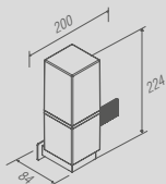
PR 0074 - Glam Porta objetos fixo
