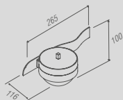
PR 0002 - Paper Porta objetos fixo
