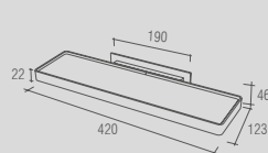
BA 0210 - Supreme Prateleira de inox
