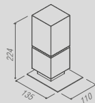
PR 0025 - Oriente Wood Porta objetos de balcão
