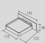
BA 0209 - Supreme Saboneteira fixa de inox
