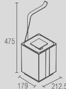
BA 0386 - Spirit Papelera de chão c/ lixeira 5L
