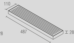
BA 0524 - Soho Prateleira inox
