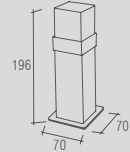
BA 0147 - Spirit Porta objetos de balcão
