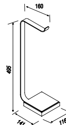
Soho - BA0500 Papeleira de chão
