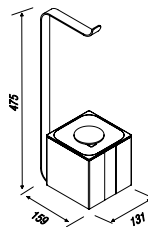
Soho - BA 0502 Papeleira de chão c/ Lixeira 1,5l
