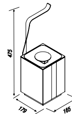
Soho - BA 0503 Papeleira de chão c/ Lixeira 5l
